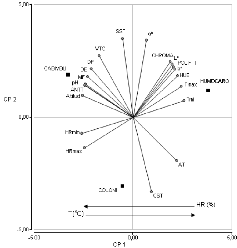
Figura 1. Análisis de los componentes principales (ACP) de las variables físicas (MF: masa fresca, DE: diámetro ecuatorial, DP: diámetro polar, CST: consistencia, índices de color: L*, a*, b*, hue, chroma) y variables químicas (SST: Sólidos solubles totales, pH, ANTT: acidez total titulable, VTC: vitamina C, ANTT: antocianinas totales, POLIF.T: polifenoles totales) en fresas cultivar Capitola y su relación con el clima (altitud, temperatura y humedad relativa) en Humocaró Bajo, Páramo de Cabimbú y Colonia Tovar de los estados Lara, Trujillo y Aragua, respectivamente
